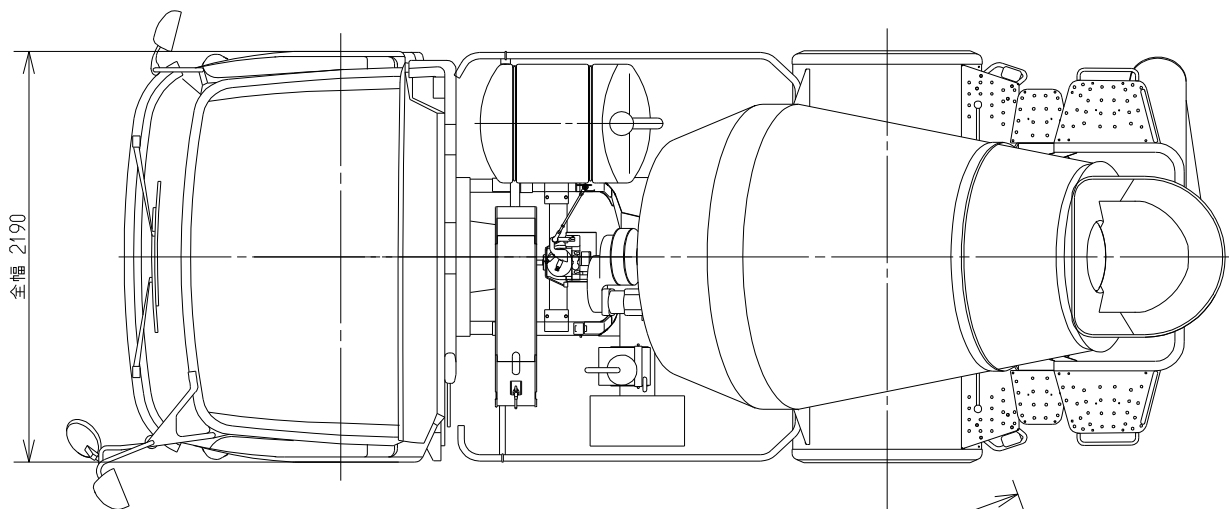
4t車サイズ表【目安】
