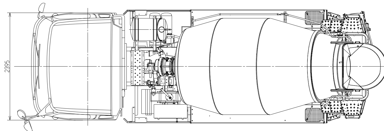
10t車低床5m 3 サイズ表【目安】
