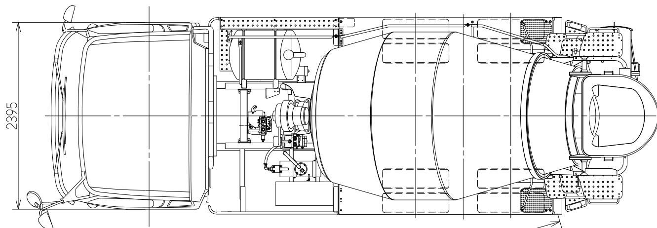
10t車低床サイズ表【目安】
