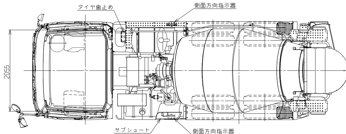
10t車高床サイズ表【目安】
