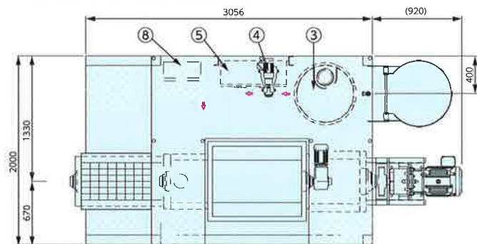
外形寸法図（ご参考）
